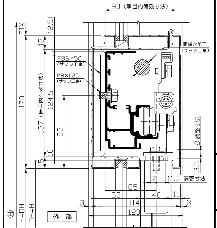
EBベースのフラットバー納り (参考例)
