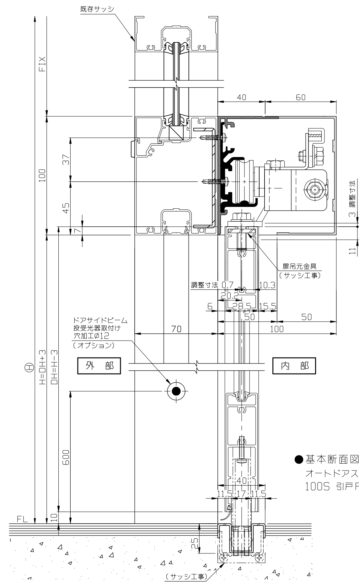
●基本断面図 オートドアスタンダードスリム 100S ドア枠
